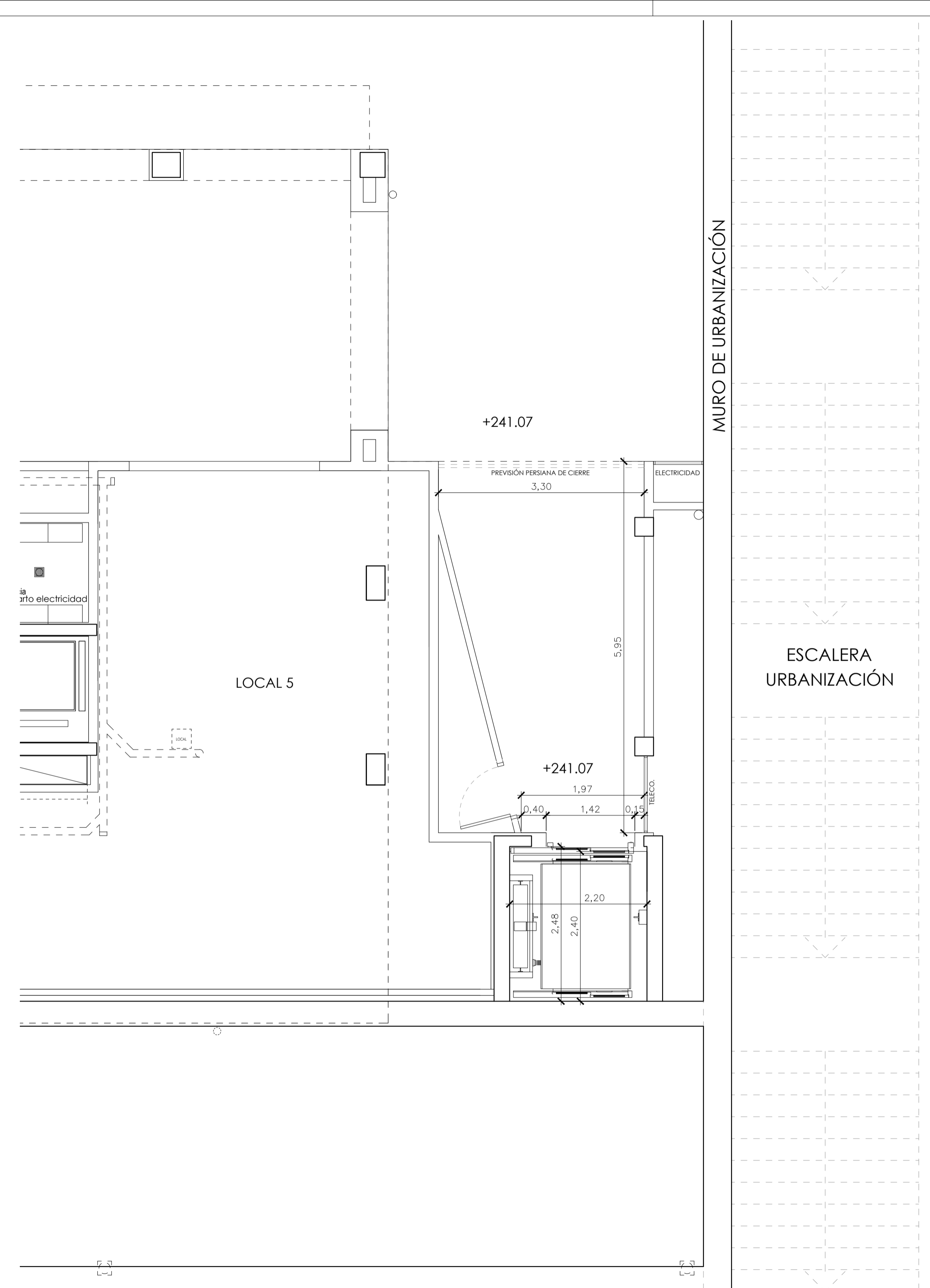
PLANTA BAJA ACOTADA/ BEHEKO SOLAIRU KOTATUA
