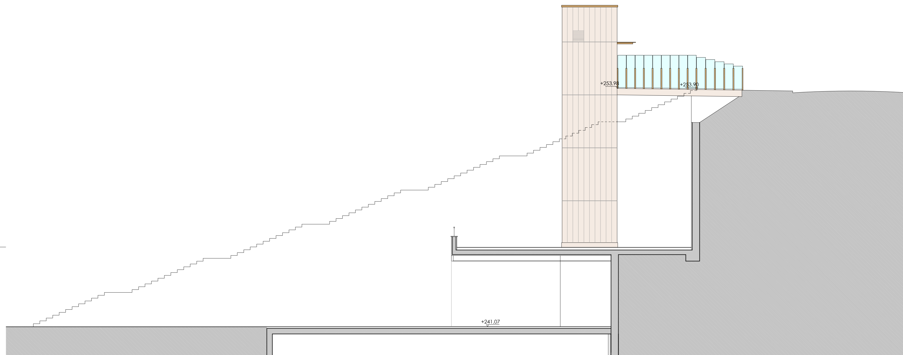
ALZADO NORTE / IPARRALDEKO ALTXAERA
