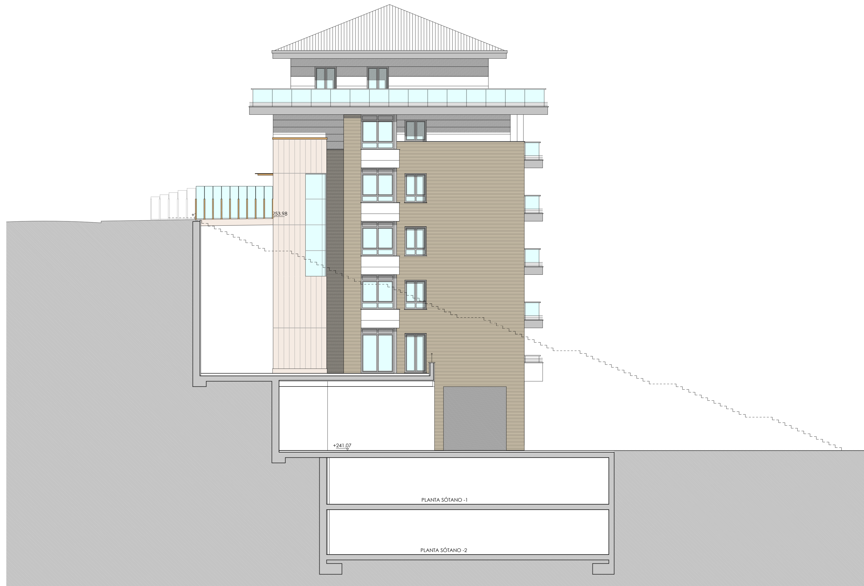
ALZADO SUR / HEGOALDEKO ALTXAERA
