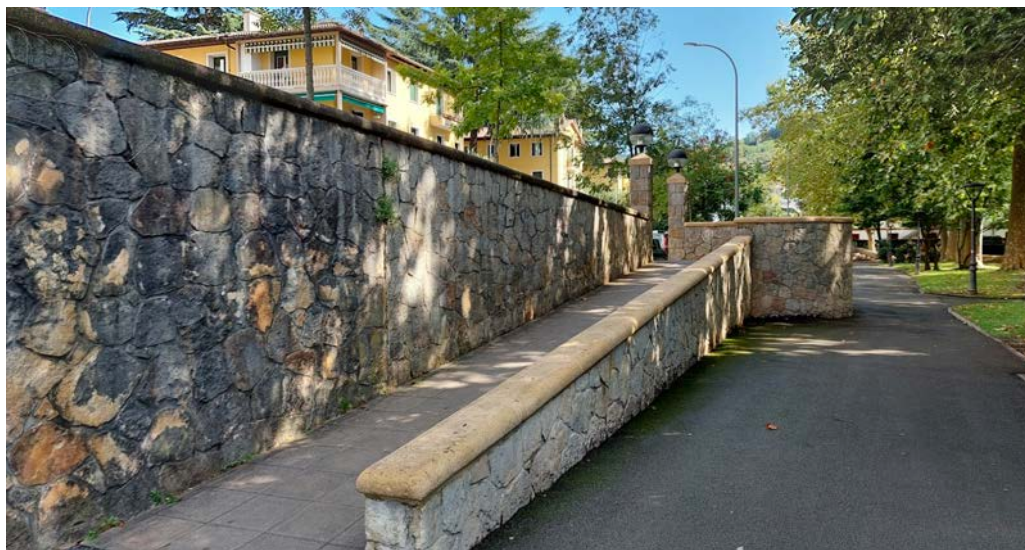
Arrapalek atsedean hartzeko eskailera-buruak izan behar dituzte, eta zenbat eta malda handiagoa izan, orduan eta laburragoak izango dira hauen arteko tarteak. Asko dira tarte horizontalik gabeko arrapalak, Ordiziako hau, esaterako.
